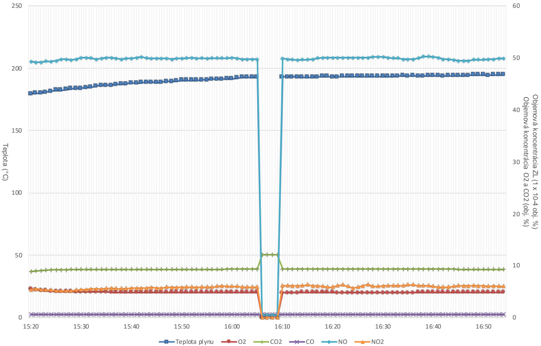
Grafický záznam priebehu merania emisií ZL
